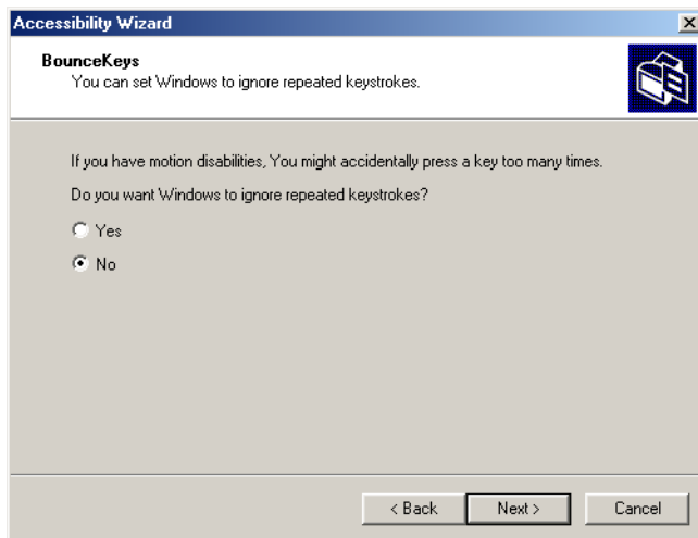
Fig. 24.31 BounceKeys dialog.
